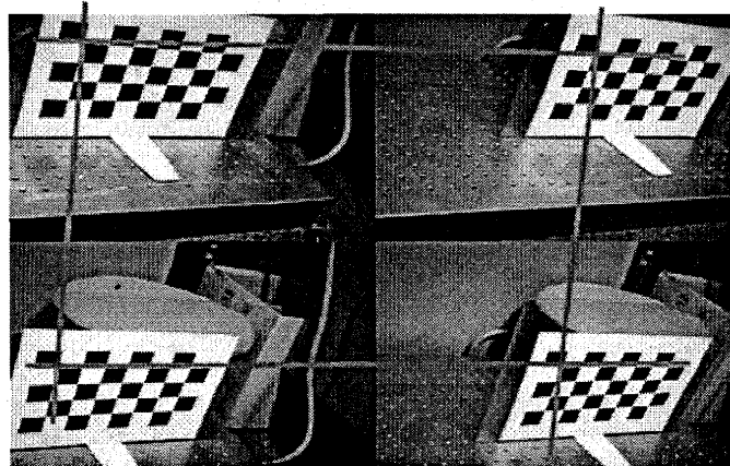
Fig. 7. Input image
